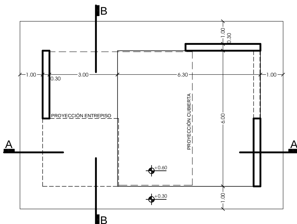
PLANTA ESC 1:100
