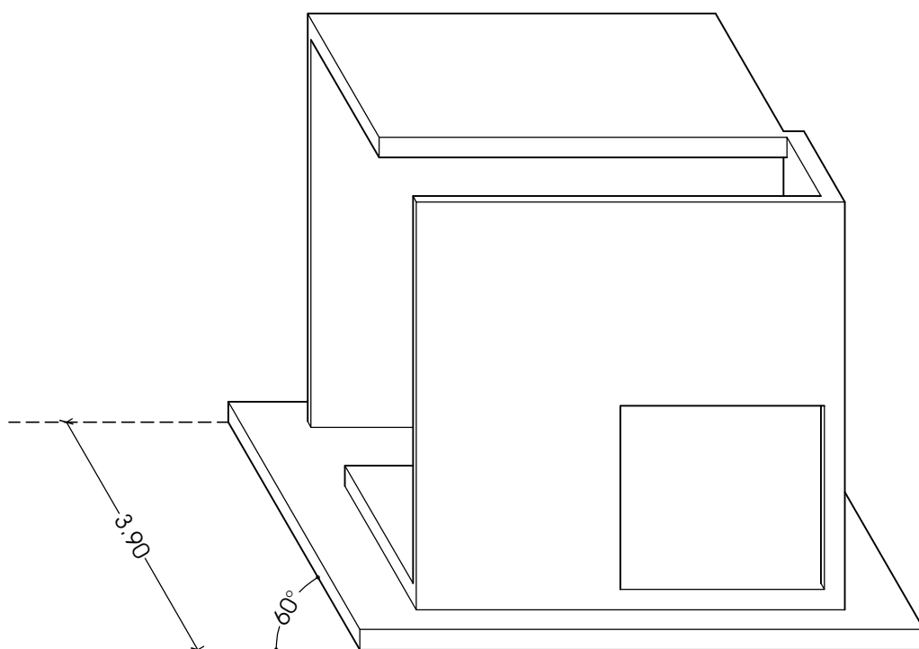
PERSPECTIVA CABALLERA DE FRENTE A 60° ESC 1:100
