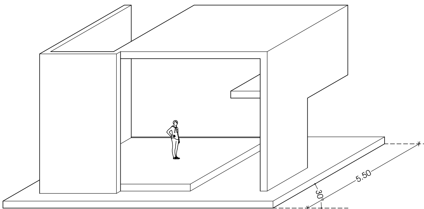
PERSPECTIVA CABALLERA DE FRENTE A 30° ESC 1:100
