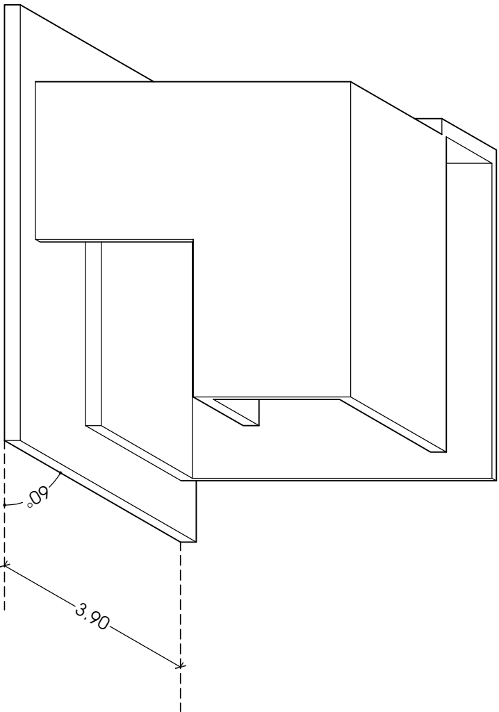
PERSPECTIVA CABALLERA DE FRENTE A 60° ESC 1:100 Aunque la profundidad real es de: 11.60, en esta perspectiva se dibuja sólo 1/3 de la dimensión: 3.90.
