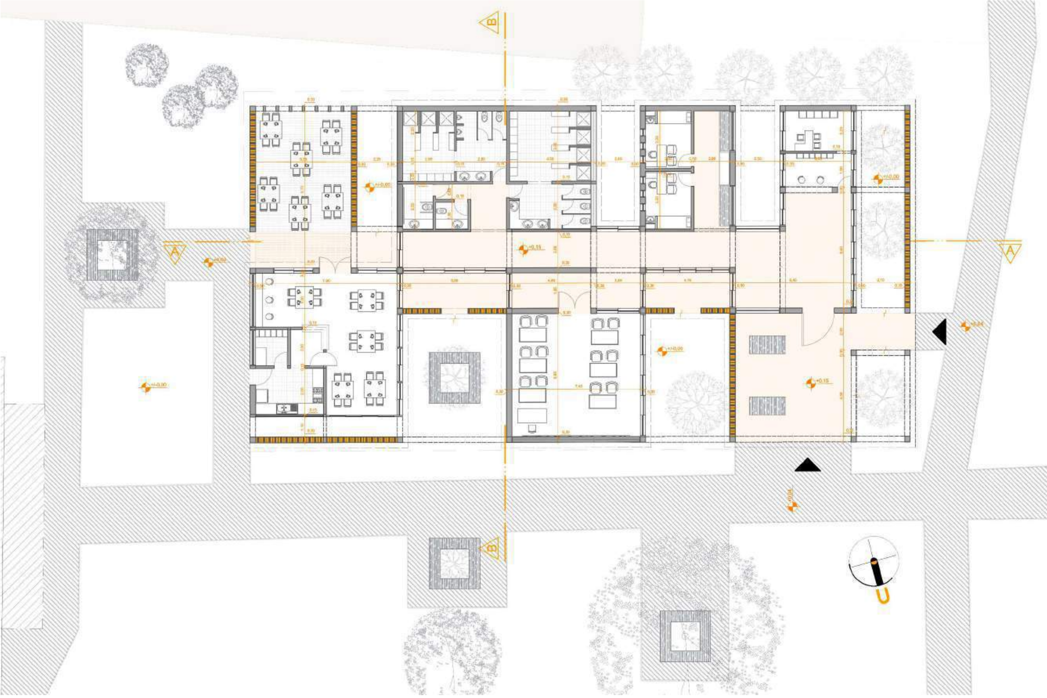
PLANTA ESC: 100
