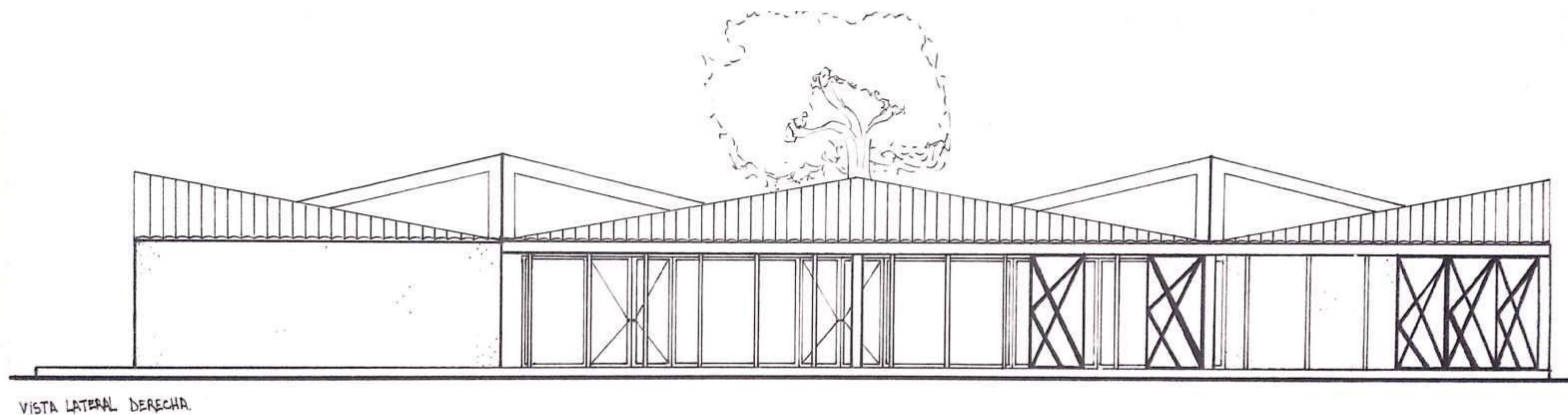
FACHADA A
