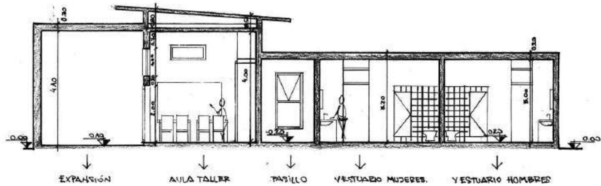
CORTE A-A
