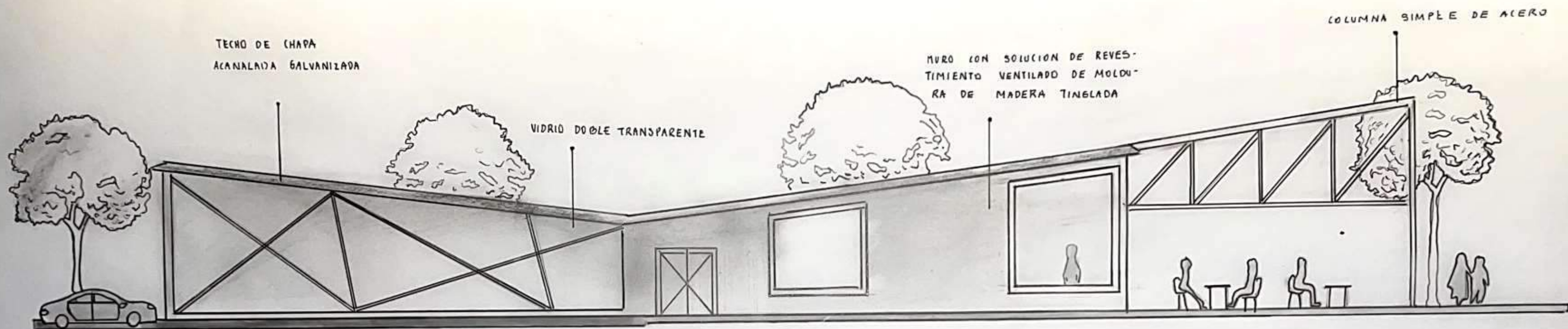
FACHADA NOROESTE
