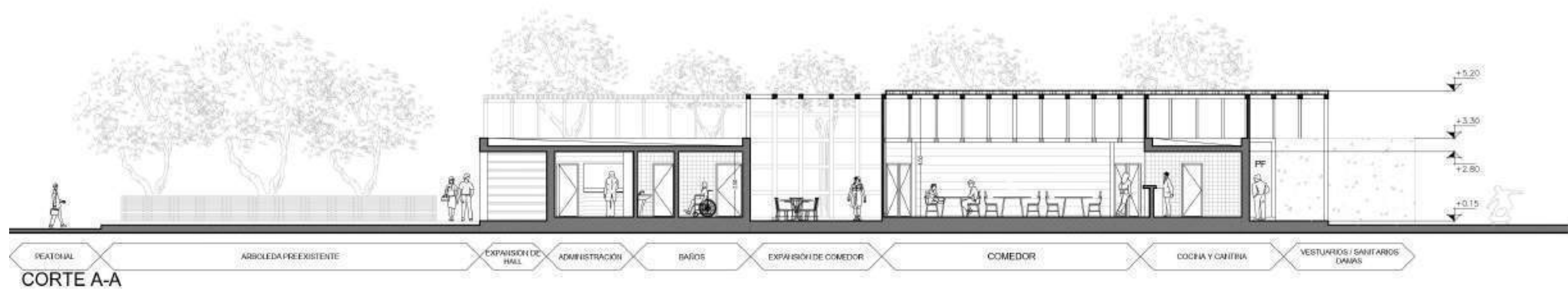
CORTE A/A
