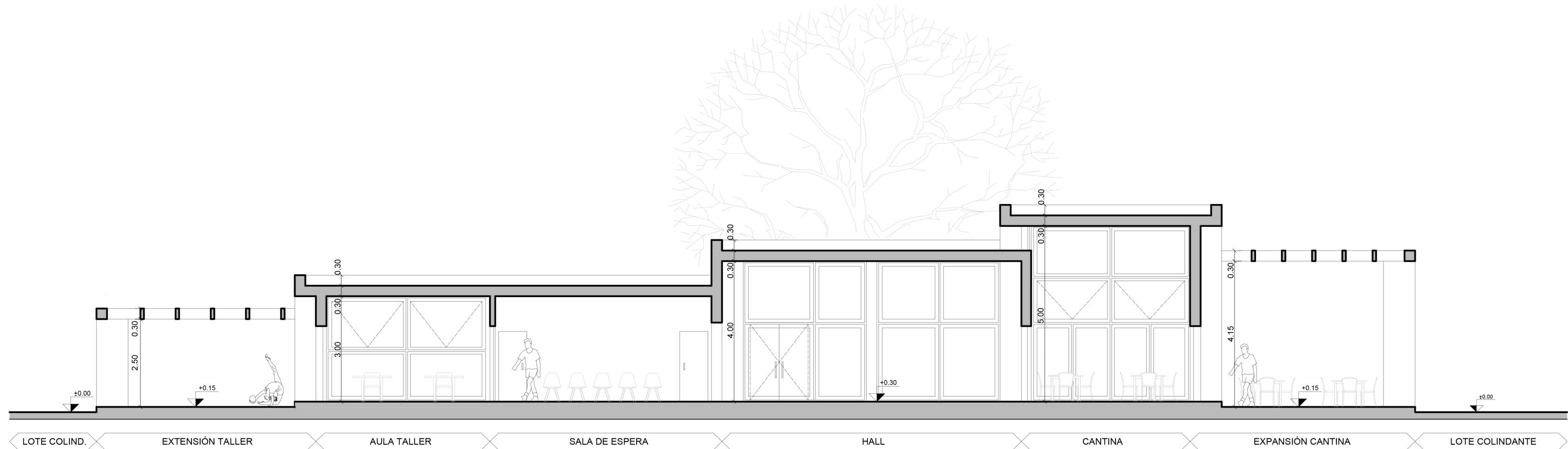
CORTE A-B
