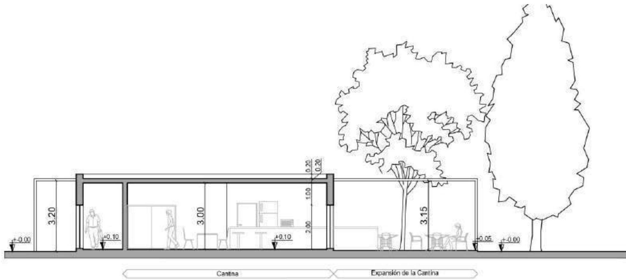
Corte C-D
