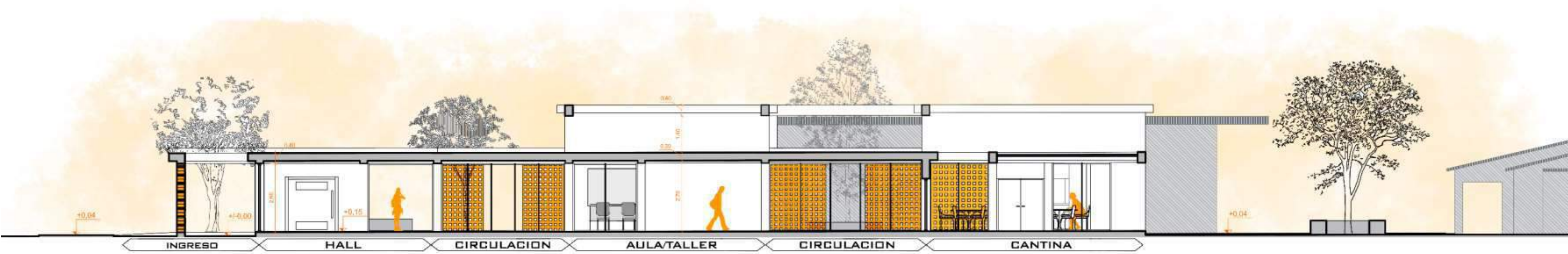
CORTE A/A
