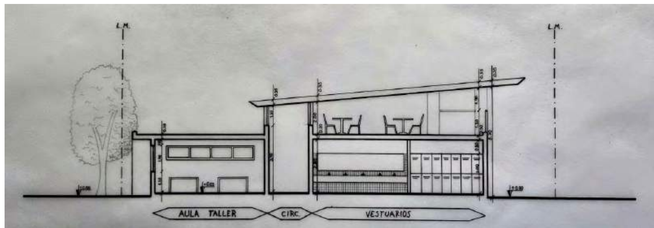
CORTE B/B
