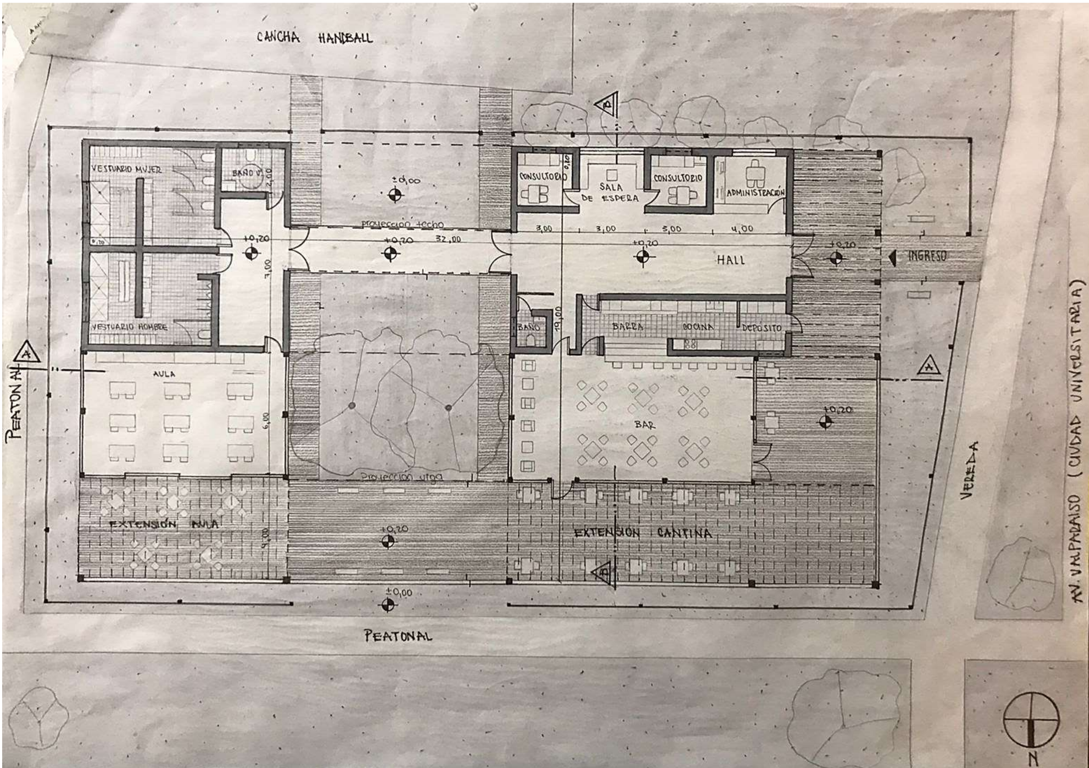
PLANTA ESC: 100
