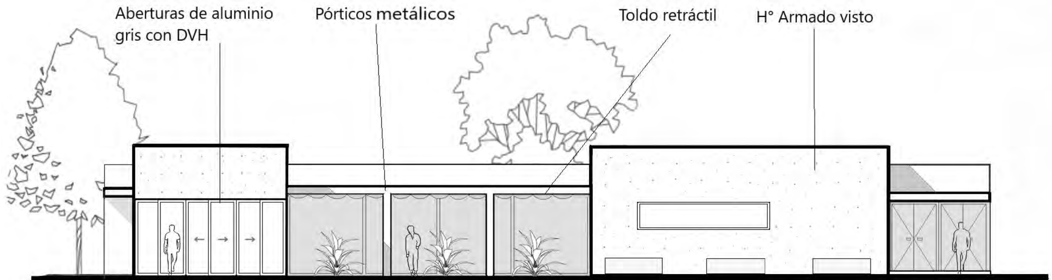
FACHADA OESTE
