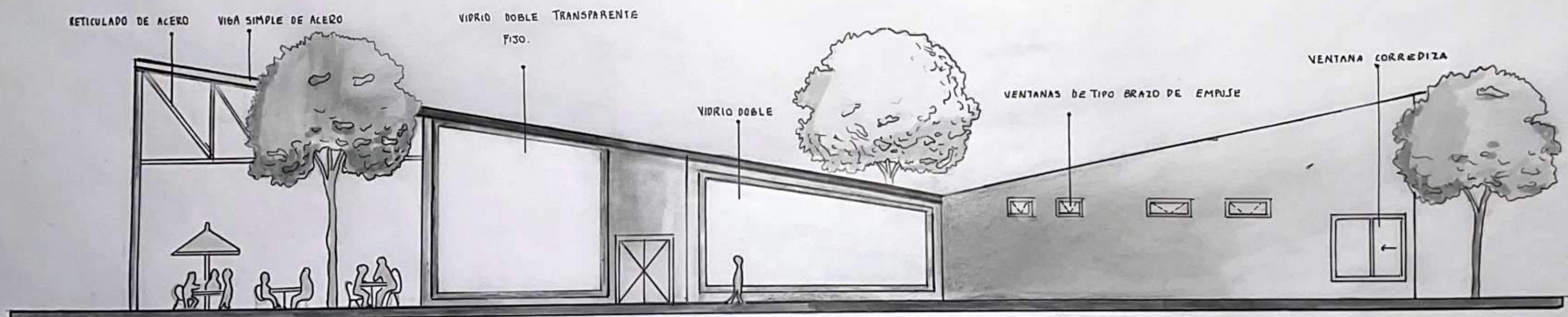
FACHADA SURESTE
