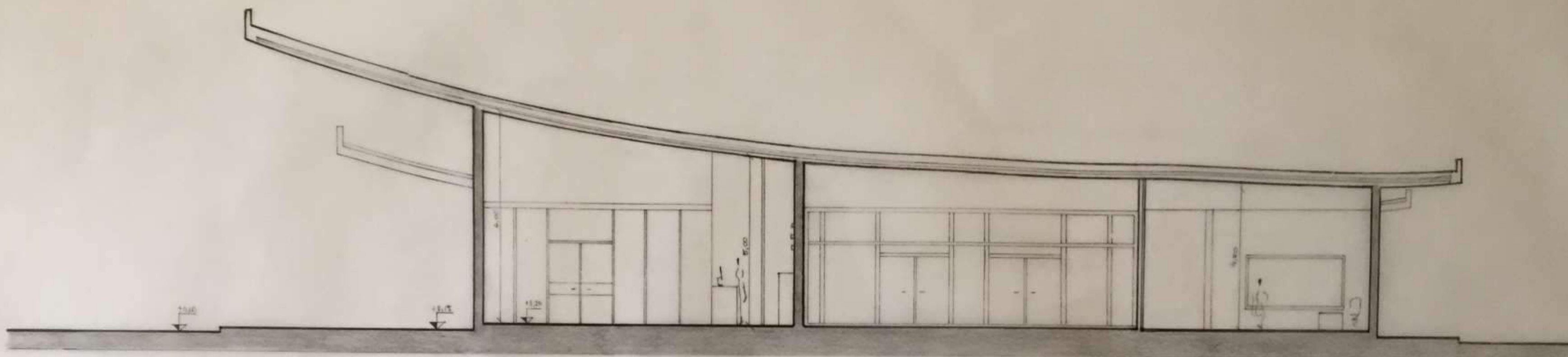
CORTE C-D
