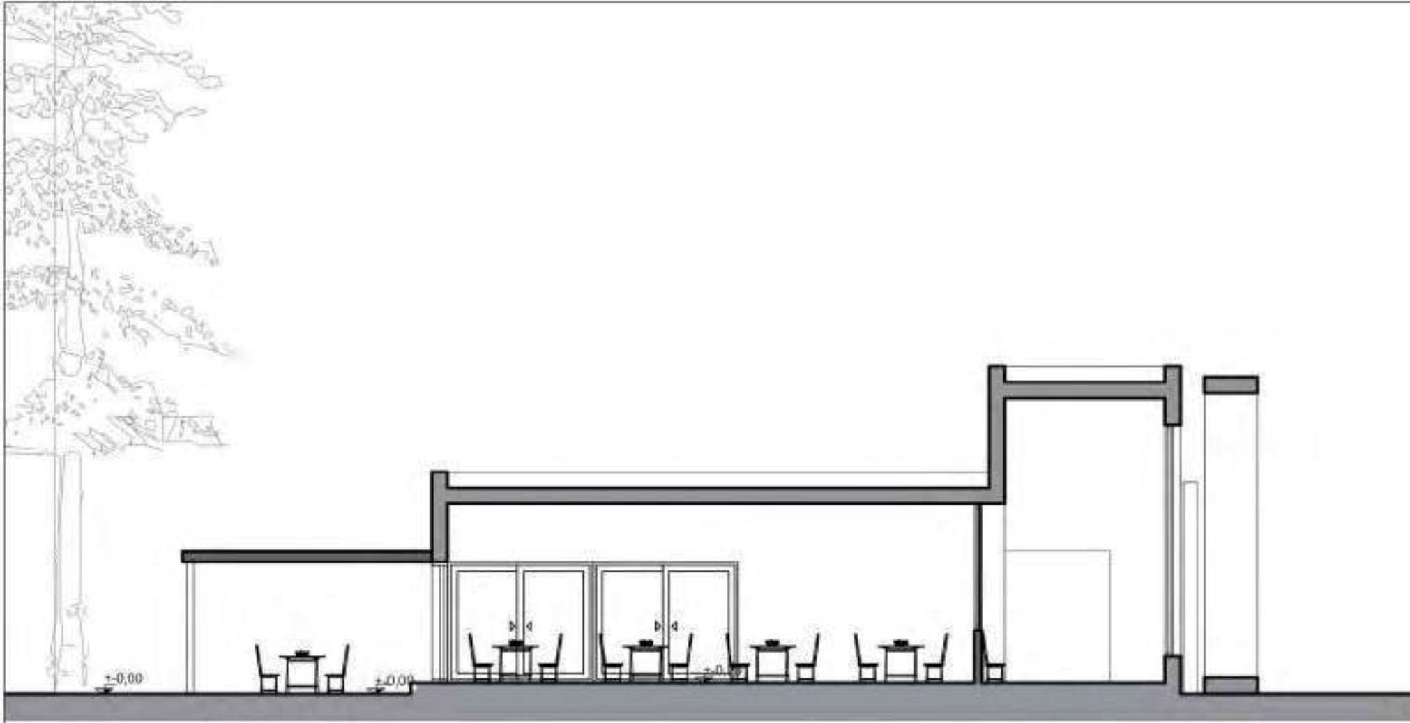
CORTE A-B
