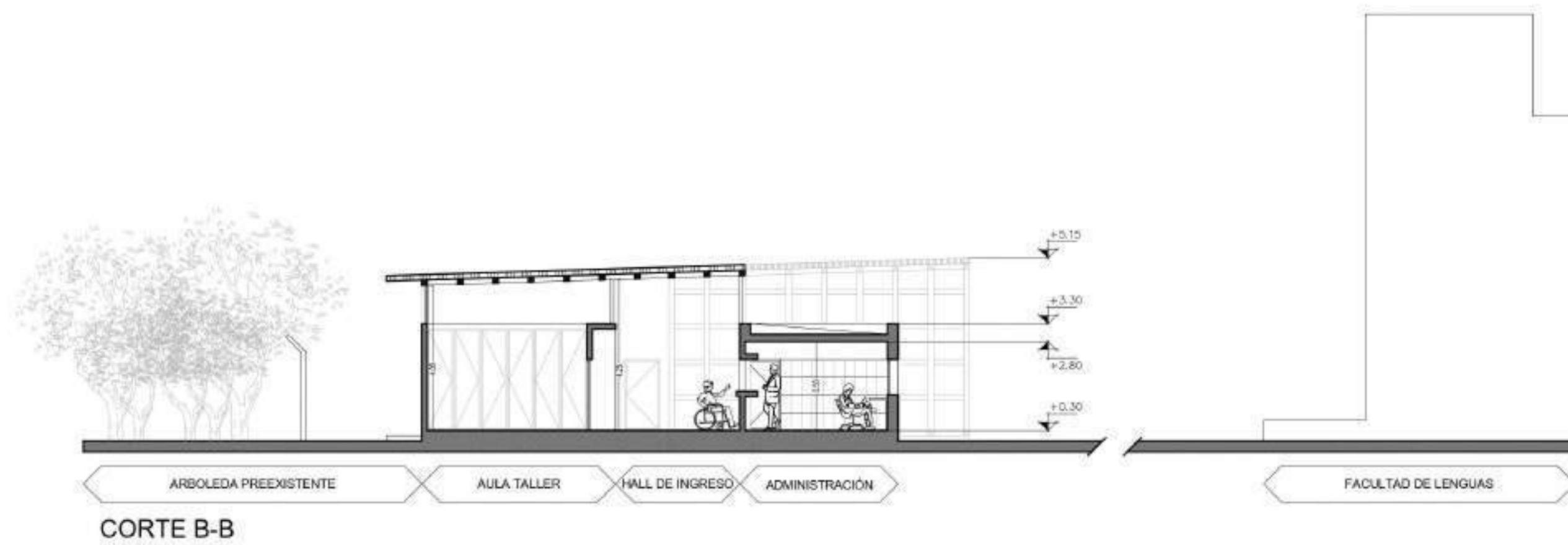
CORTE B/B
