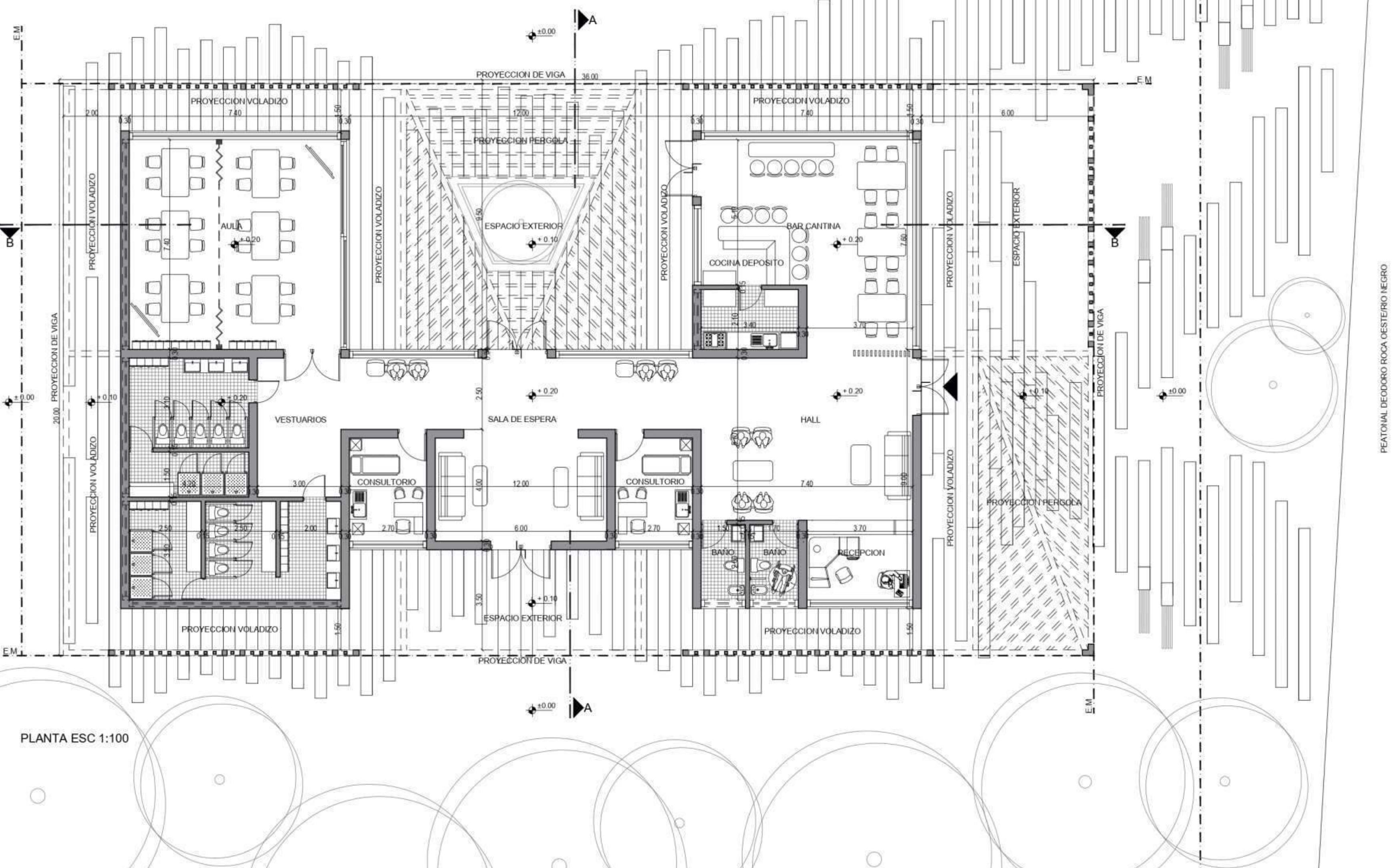
PLANTA ESC: 100
