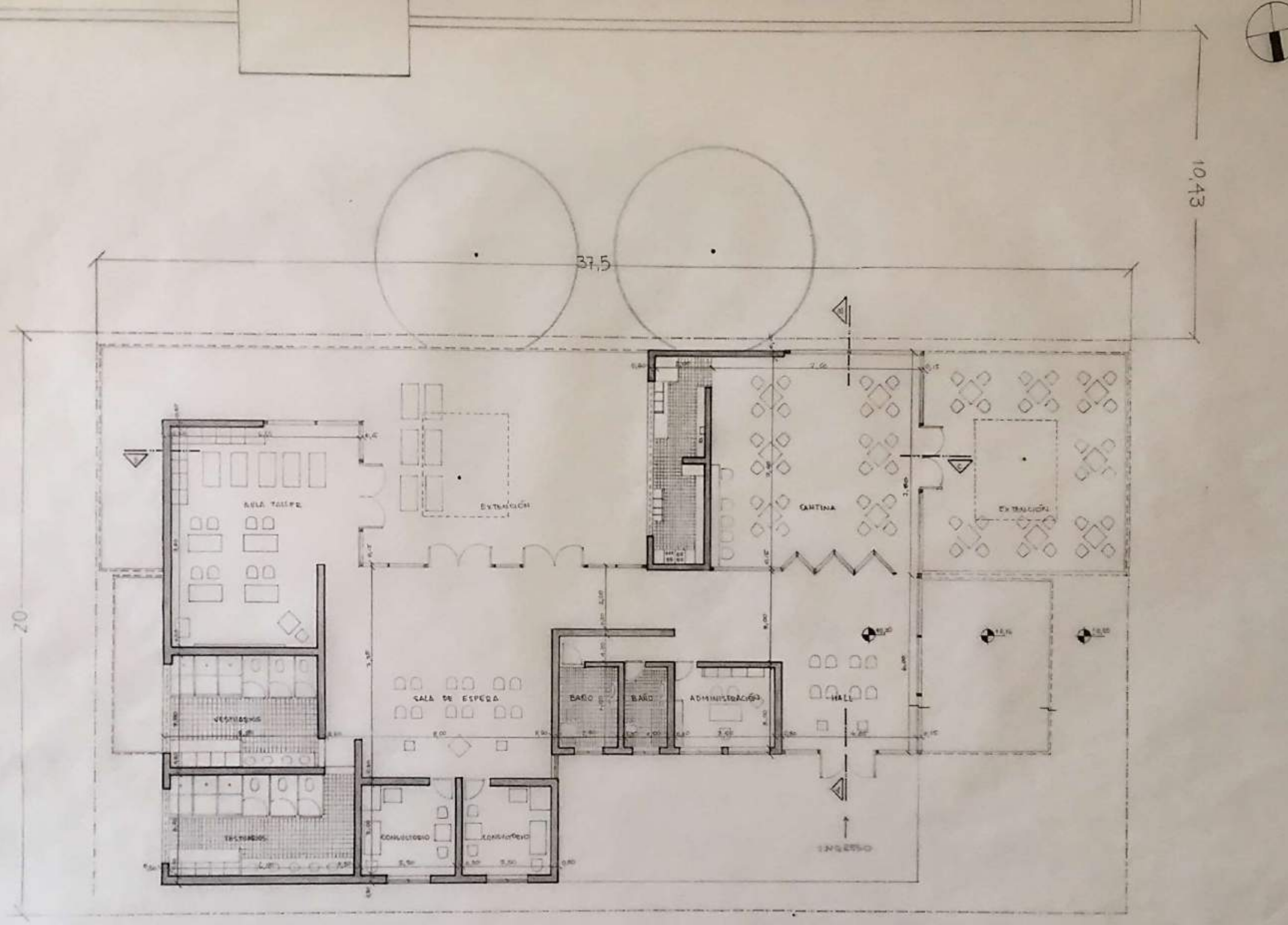
PLANTA
