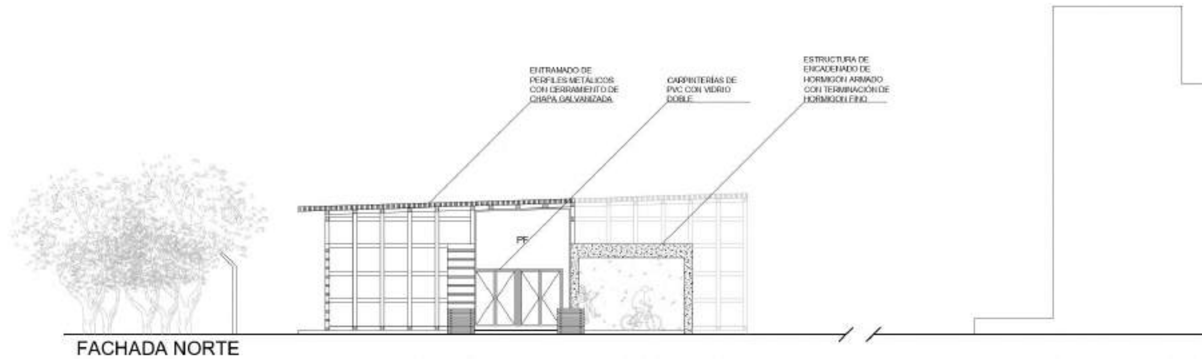
FACHADA B
