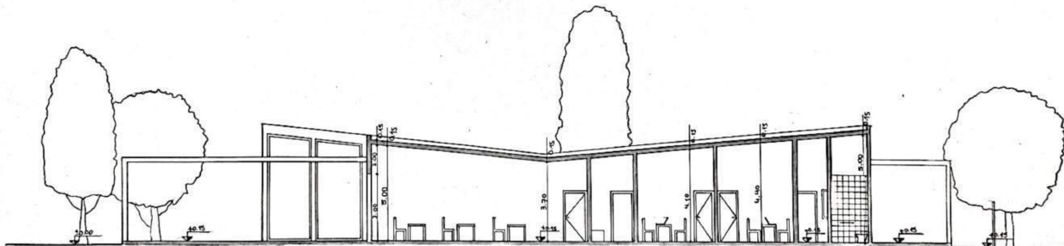
CORTE C-D
