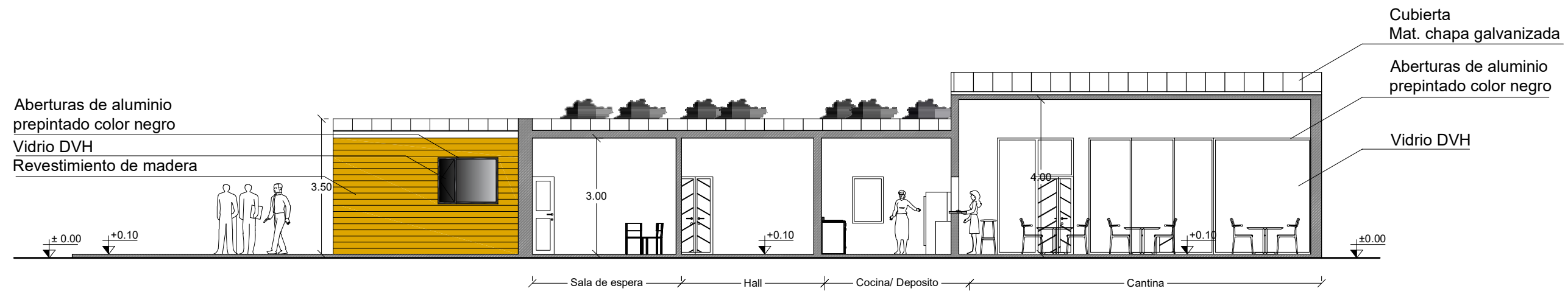
CORTE B-B
