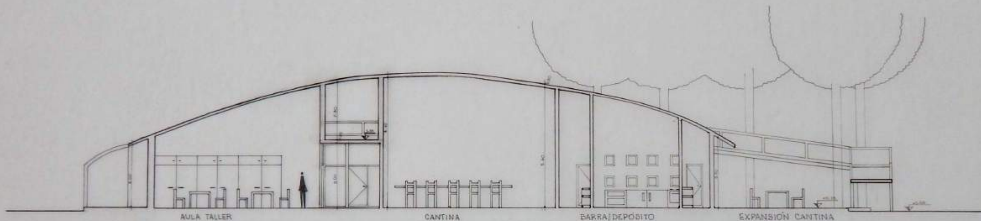
CORTE A-B
