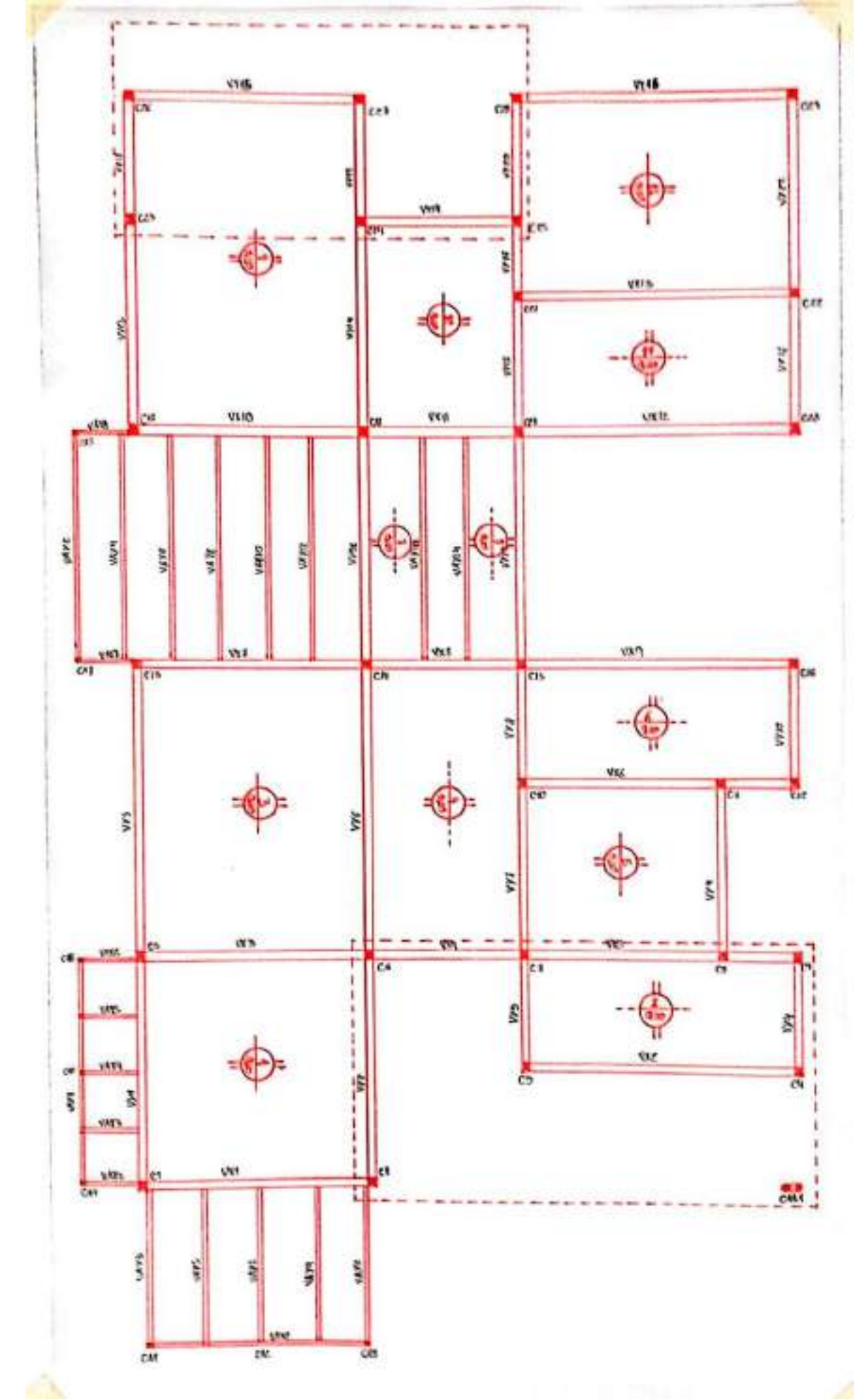
PLANTA ESTRUTURAS ESC: 100
