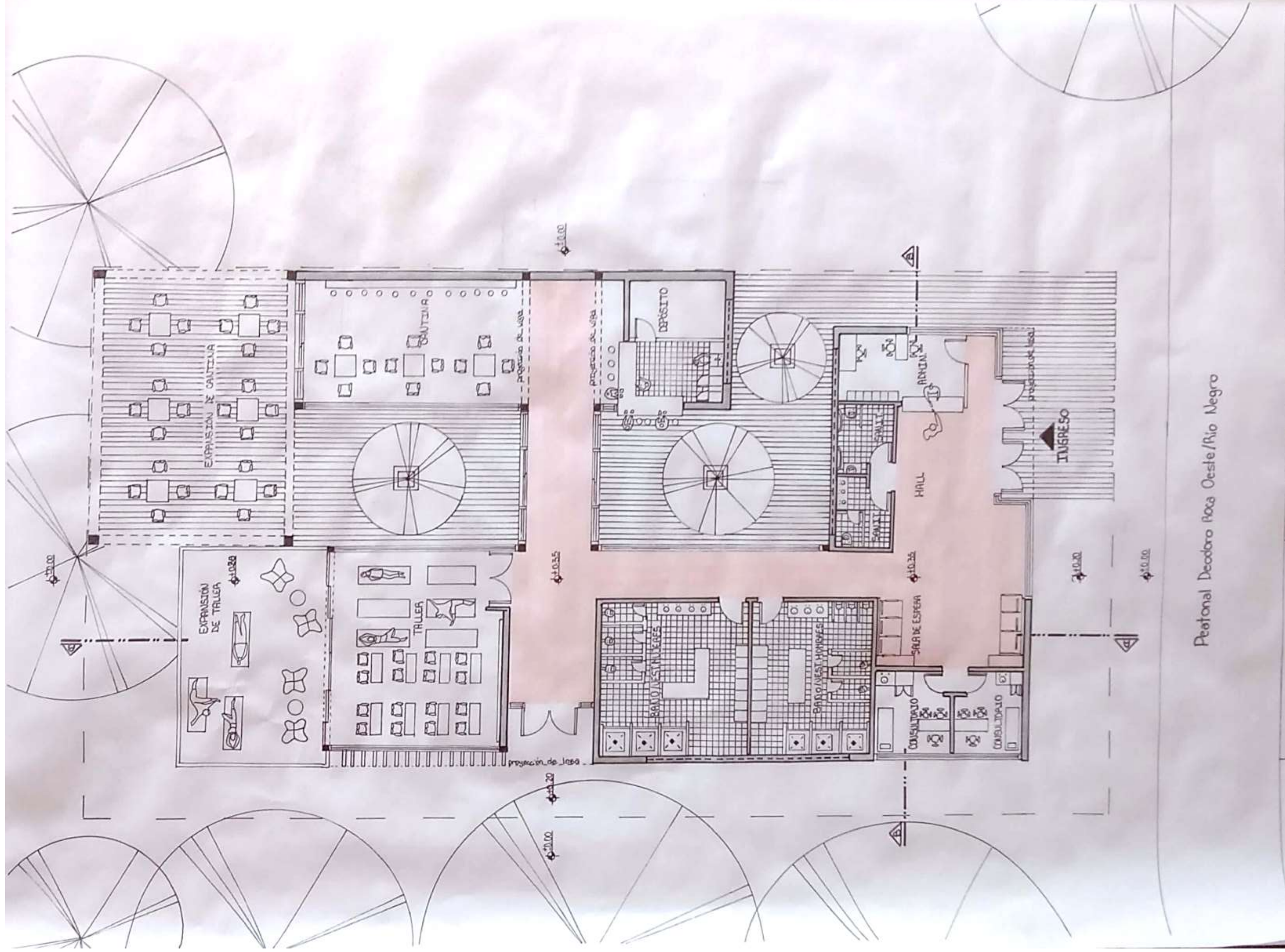
PLANTA ESC: 100
