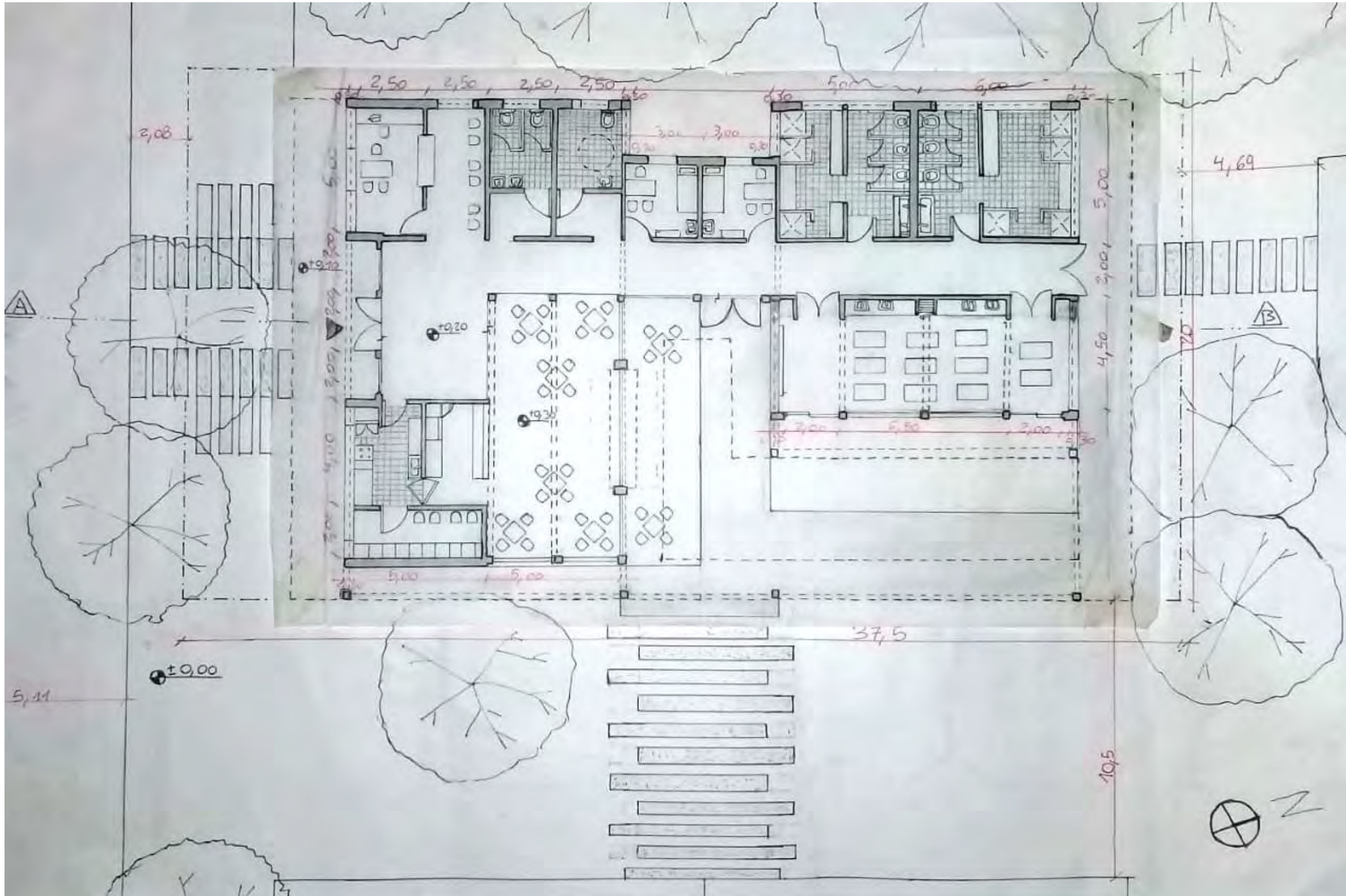
PLANTA ESC: 100
