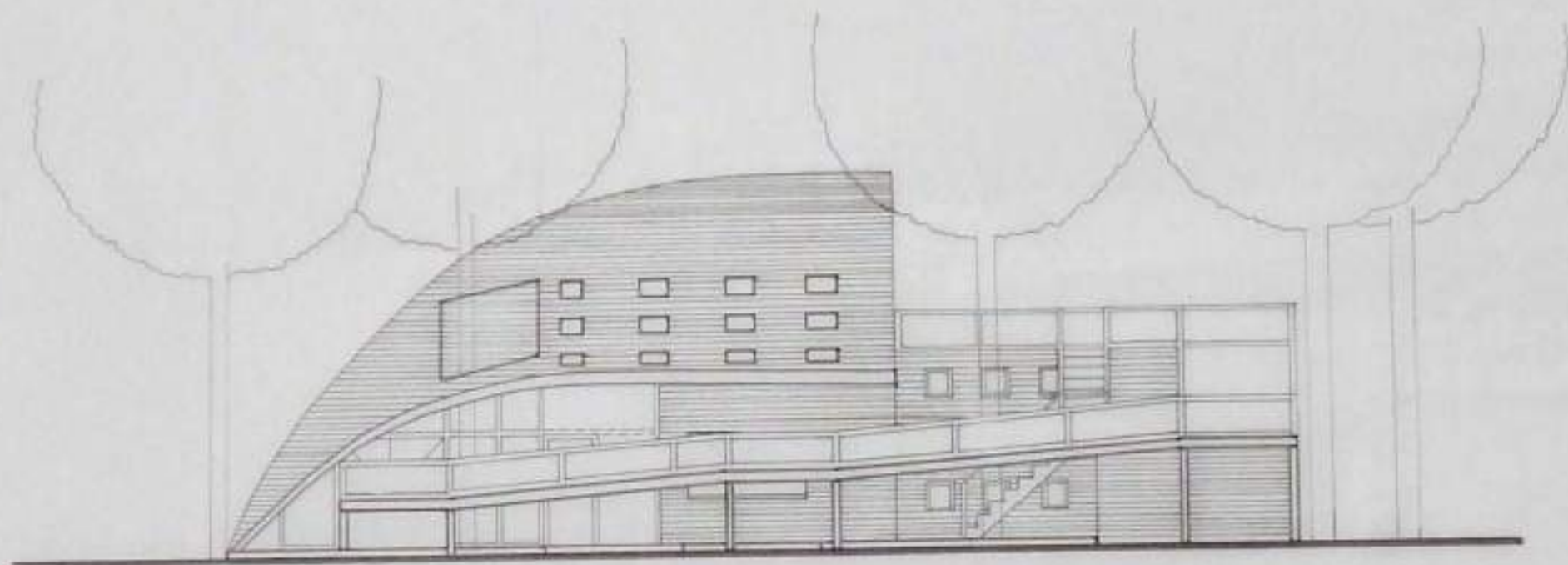
FACHADA OESTE
