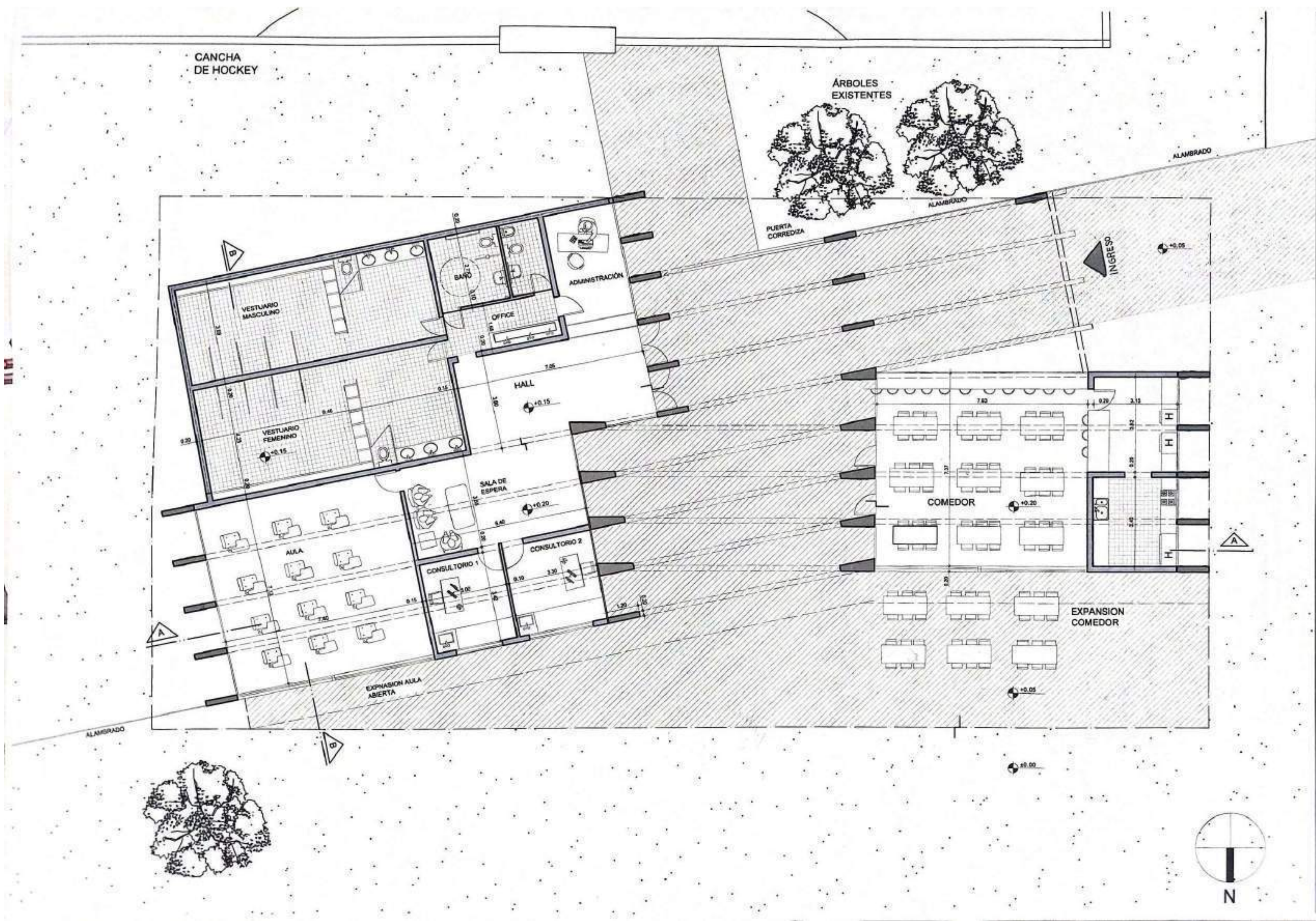
PLANTA ESC: 100
