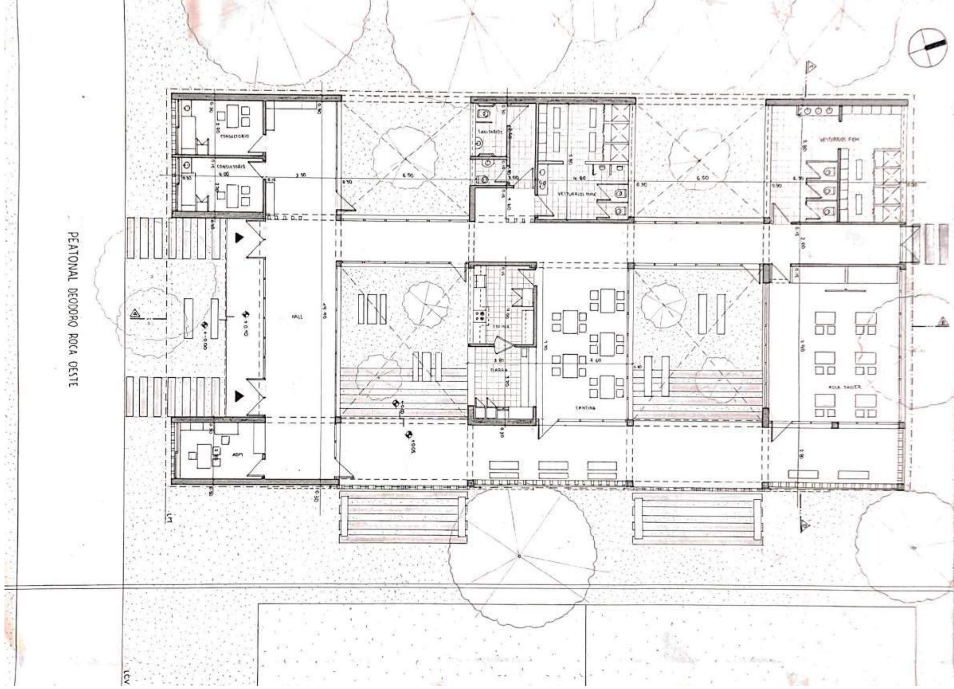
PLANTA ESC: 100
