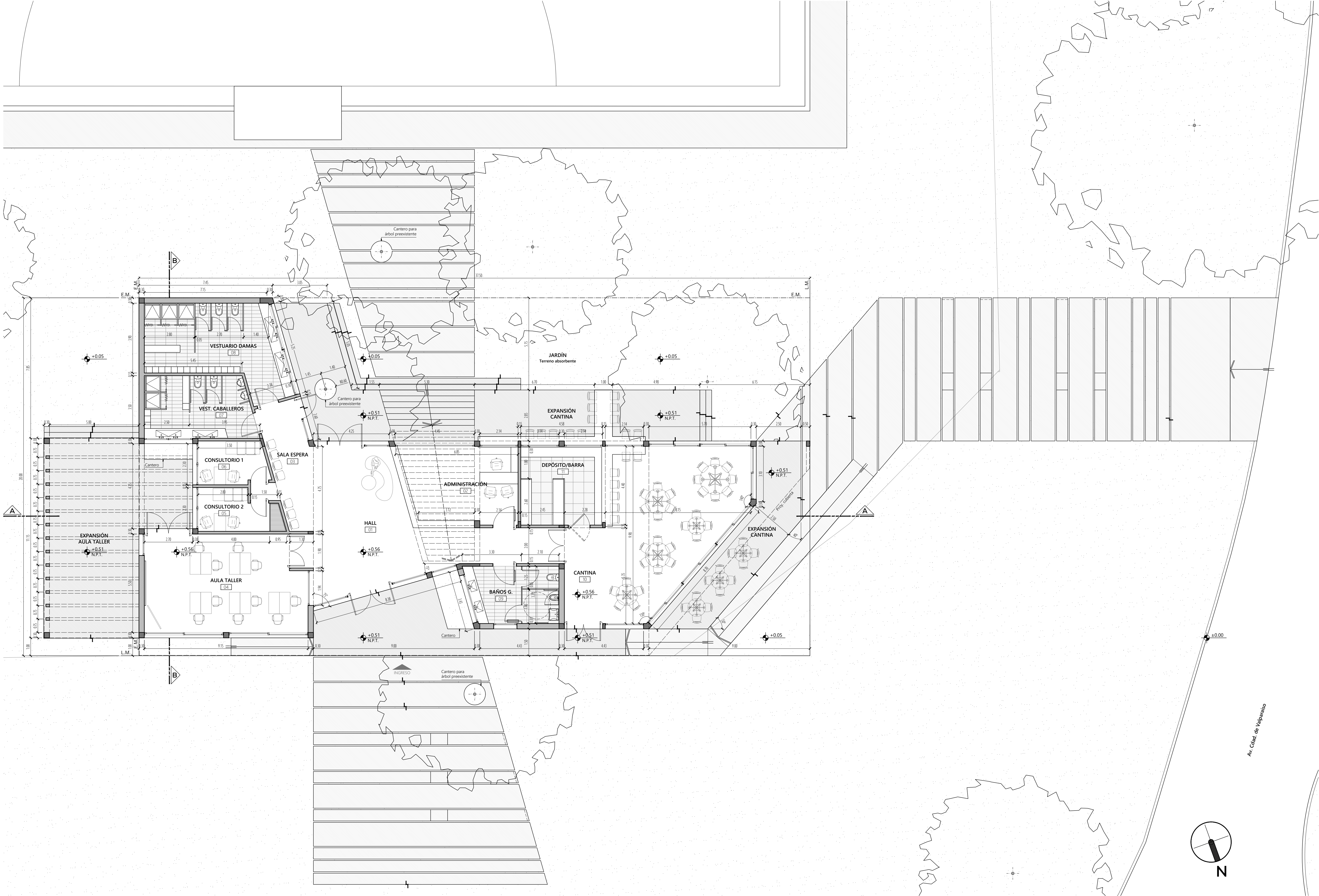
PLANTA Escala: 1:100
