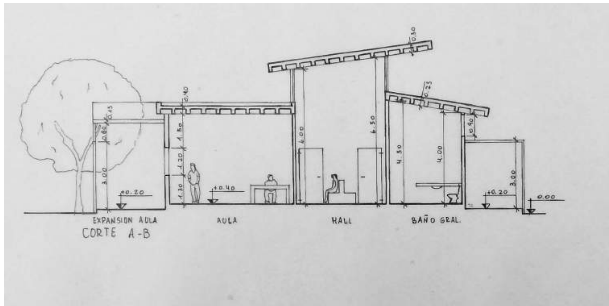
CORTE A/B
