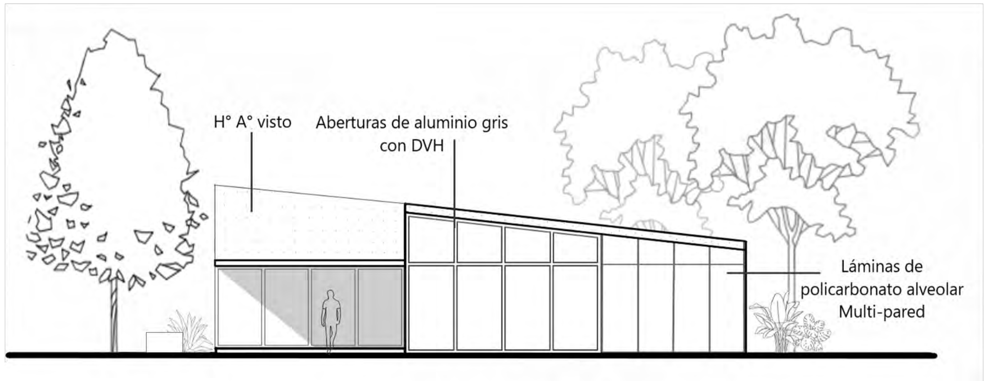
FACHADA SUR
