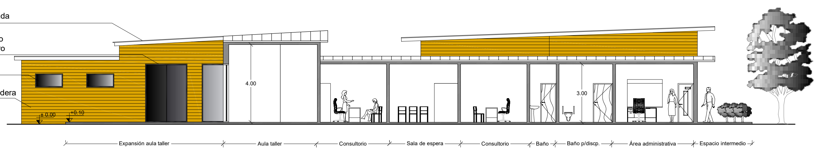
CORTE A-A
