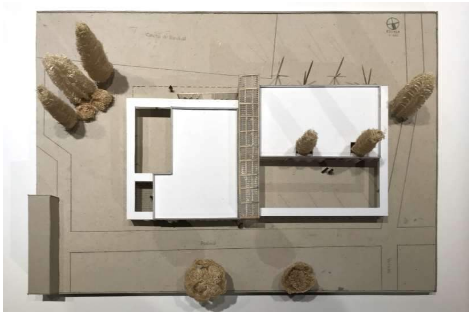
VISTA SUPERIOR
