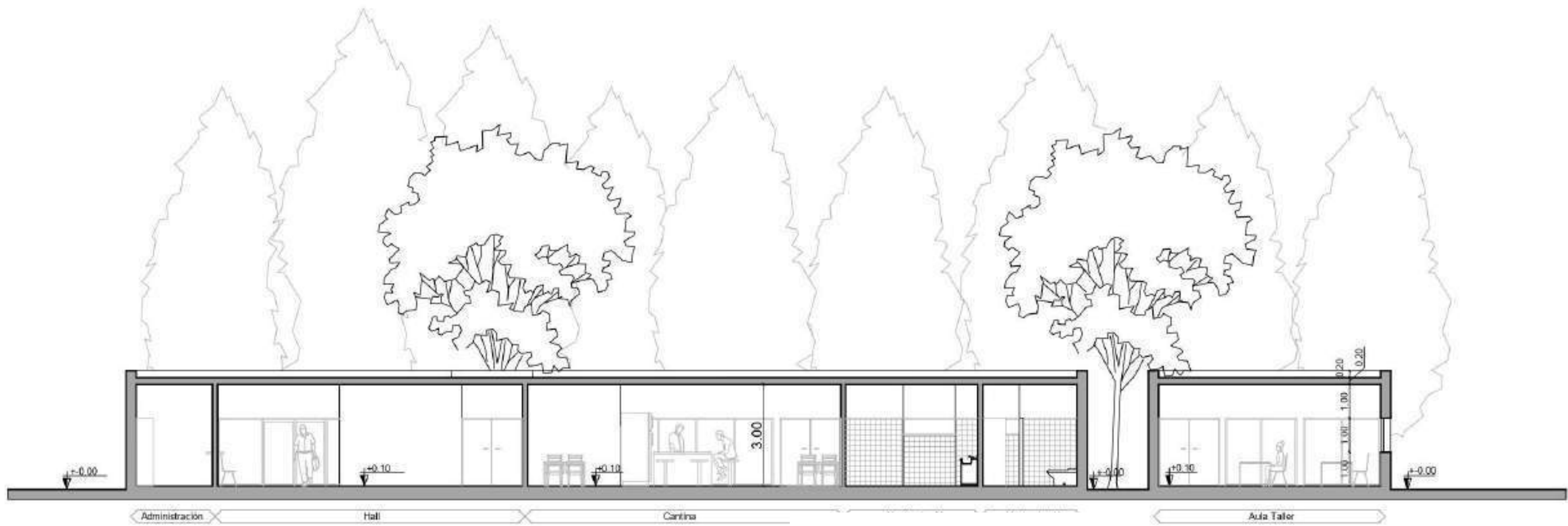
Corte A-B
