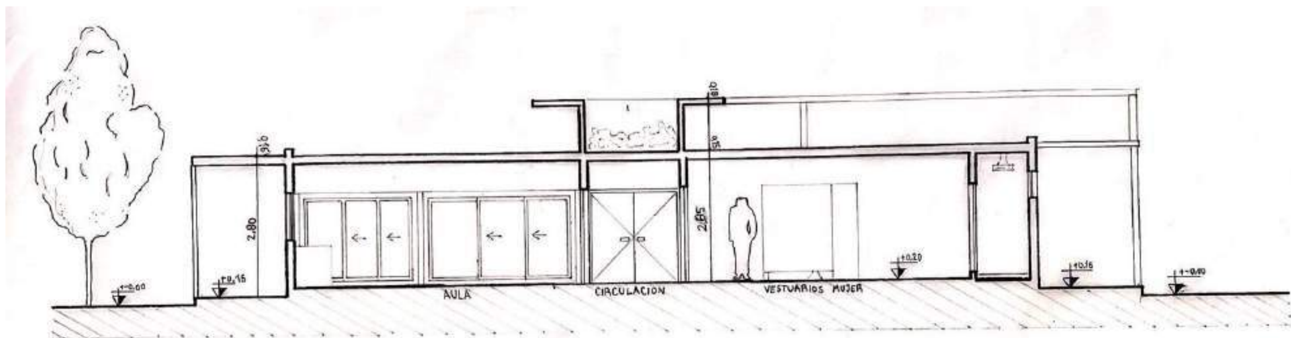
CORTE A/B
