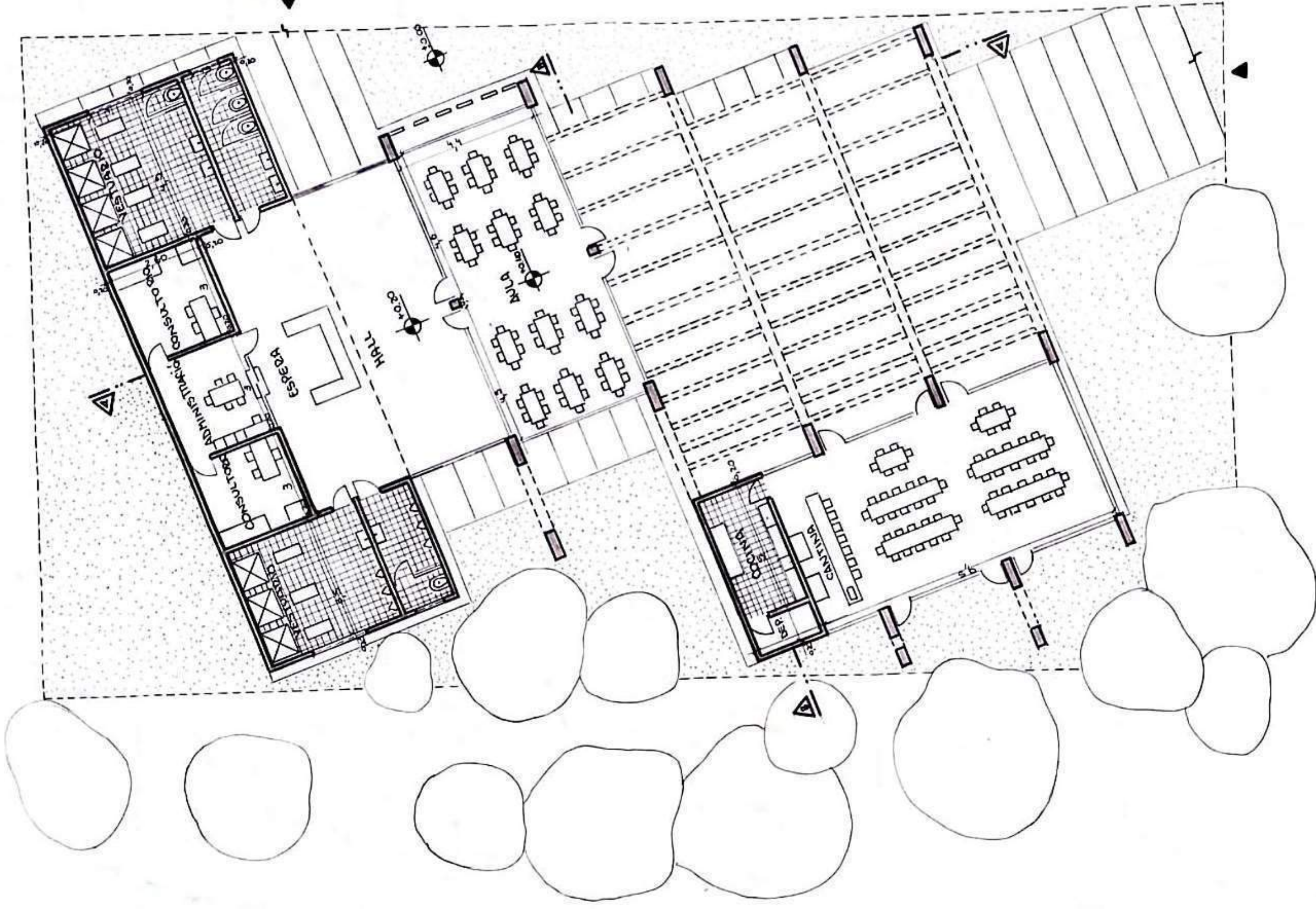
PLANTA ESC: 100
