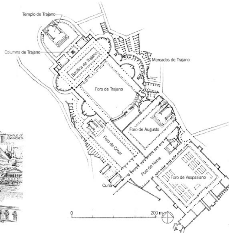
Fig. 73. Los foros imperiales: planta.
