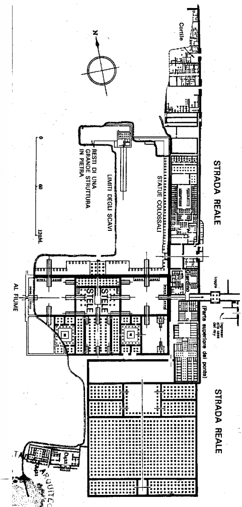
Fig. 31. Tell-el-Amarna, plano del palacio junto a la vía real.
