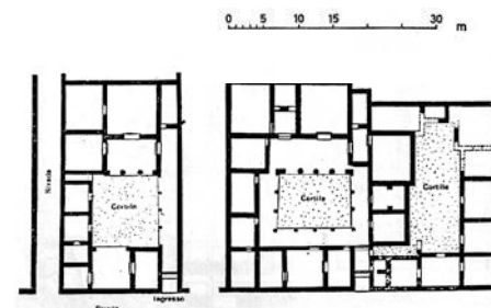
Fig. 52. Priene. Plano de dos casas típicas.
