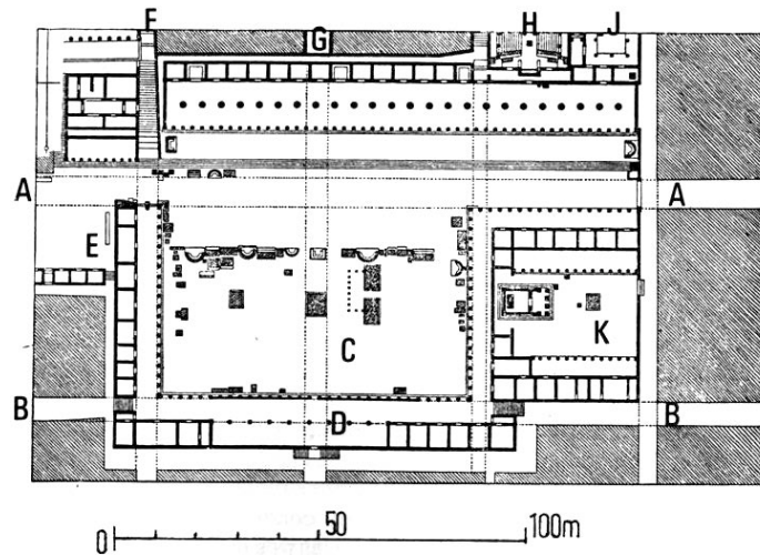
Fig. 50. Priene, plano de detalle del Agora (norte en la parte superior). A-A, calle mayor que atraviesa la ciudad de este a oeste; B-B, calle de la retícula que se prolonga por la stoa meridional, a la que se accede por unas escaleras; C, espacio del ágora principal; D, recinto porticado; E, mercado de la carne y el pescado; F, camino escalonado ortogonal en la ladera de la colina; G, la stoa norte; H, Bouleuterion; J, Prytaneion; K, Templo de Zeus.
