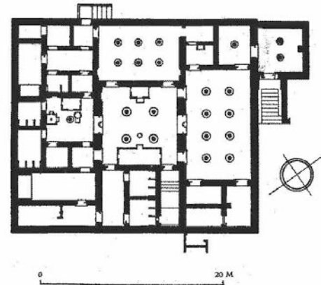
Fig. 34. Tell-el-Amarna. Plano de la casa del funcionario Nakht.
